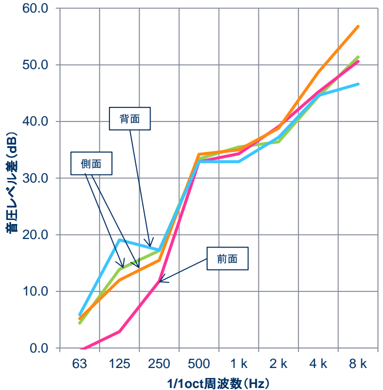
SIB設置前後における音圧レベル差
